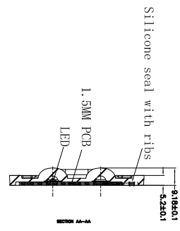
SECTION AA-AA
