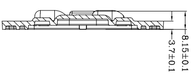
截面 A-A
