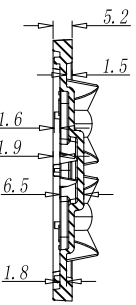
SECTION A-A
